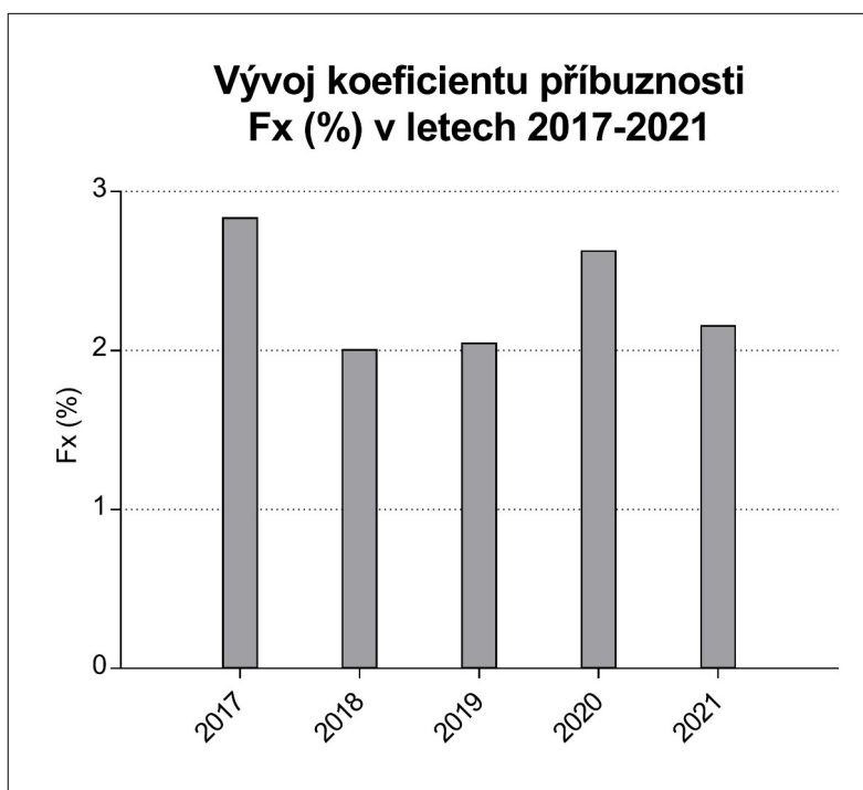
Koeficient příbuznosti Fx v letech 2017-2021
